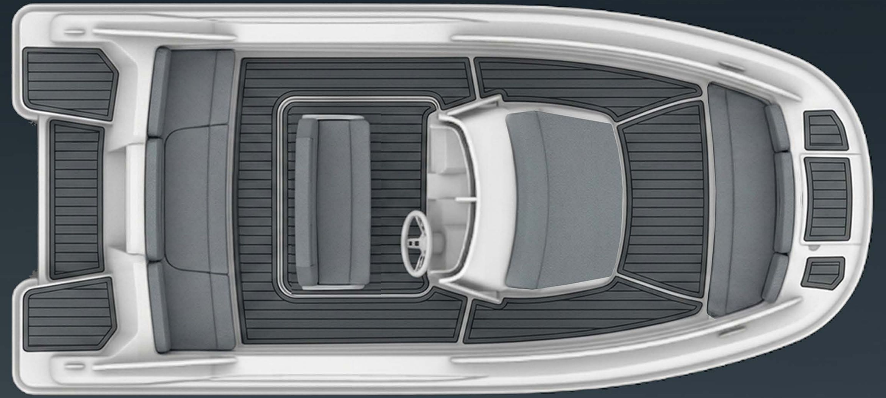
SWIFT 460 Open ÜST GÖRÜNÜŞ SWIFT 460 Open TOP VIEW
